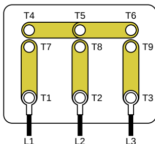
Figure 3 Conexiones de cables para un motor de 230 V
