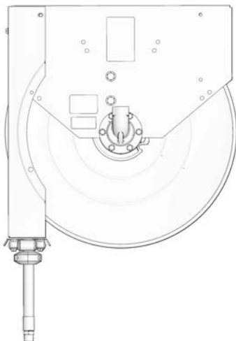
FIG. 25: Se muestra instalación suspendida
