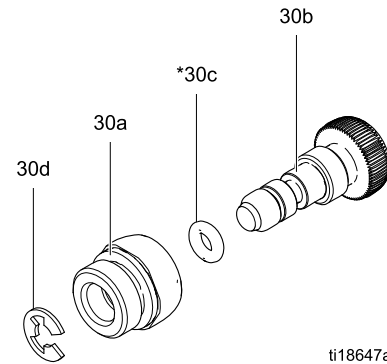
Figure 33 Válvula de ajuste de aire del abanico
