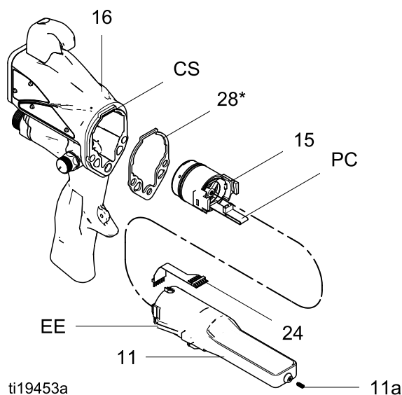
Figure 27 Fuente de alimentación
