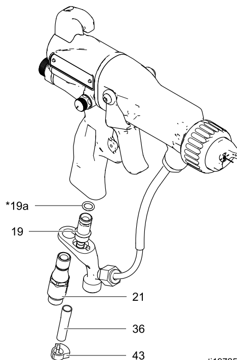
Figure 42 Accesorio de entrada de aire y válvula de escape de aire
