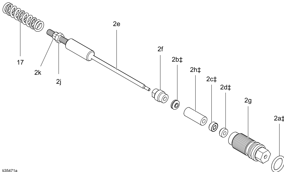
Figure 23 Varilla de empaquetadura
