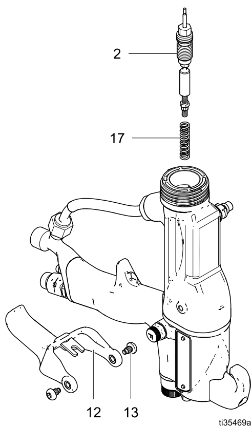
Figure 22 Desmontaje de la varilla de empaquetadura de fluido
