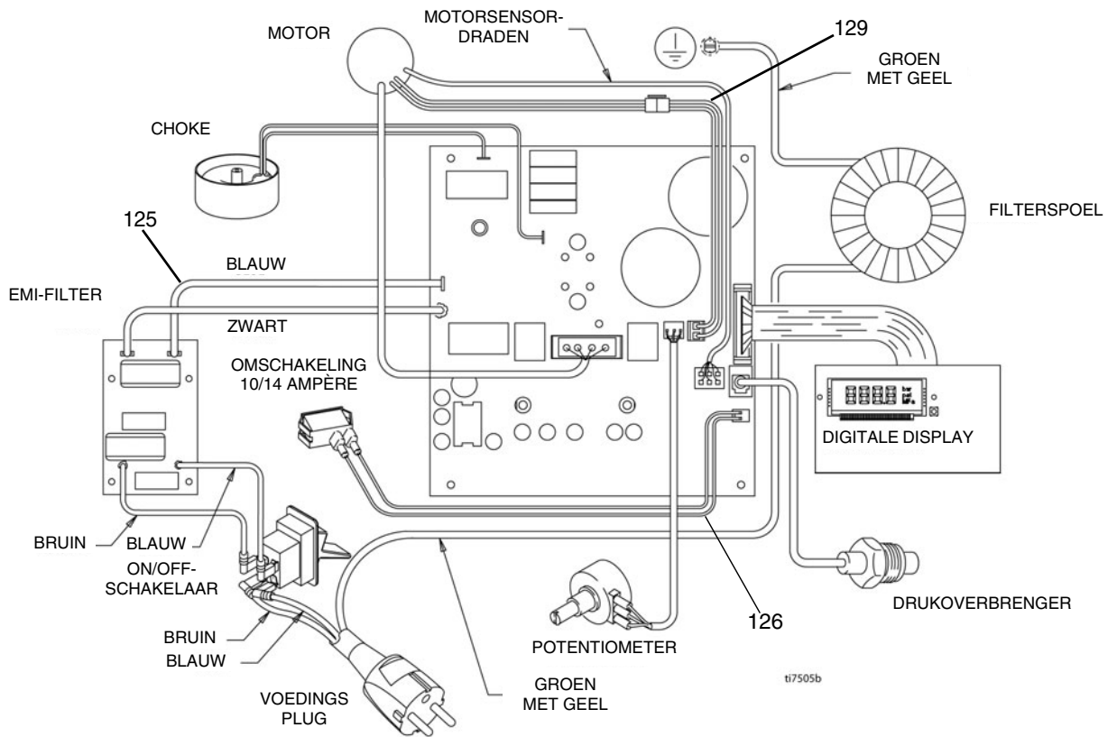
BEDRADINGSSCHEMA
