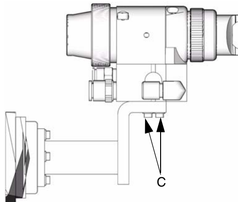
FIG. 6: Montaje de soporte estacionario
