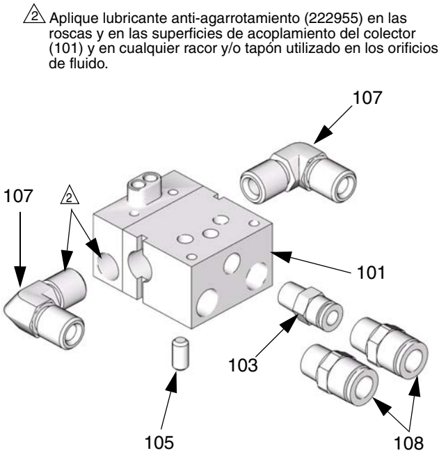
FIG. 24: Colector con orificios de fluido en el lateral
