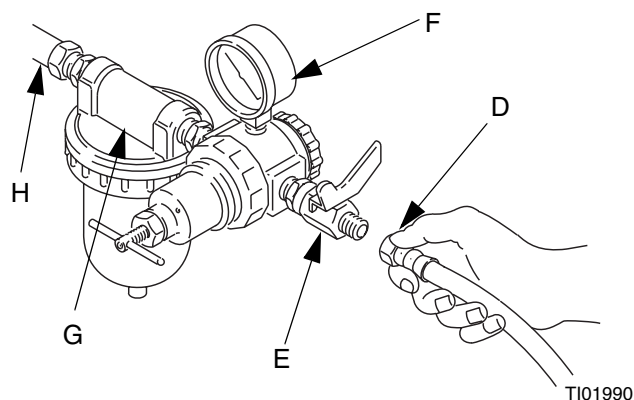
FIG. 8: Conecte las líneas de aire
