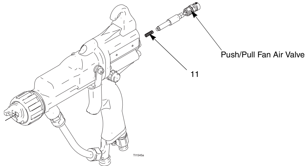
Fig. 2: Install the Push/Pull Fan Air Valve
