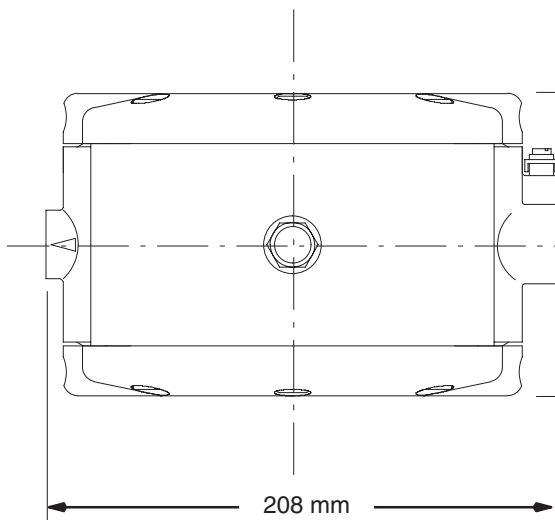
VISTA LATERAL Aluminio
