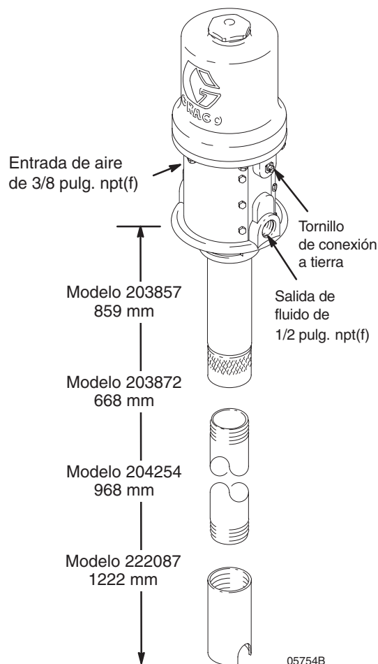
Modelo 222087, serie C depósito de 1041 litros, montaje con rosca Longitud total: 1521 mm El adaptador de rosca (118) se muestra en la página 17.
