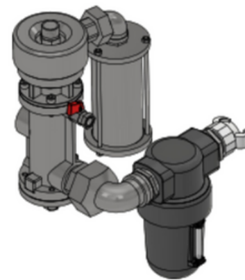
Versión con HMS
