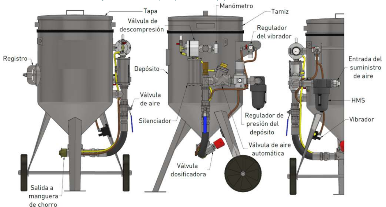
Figura 2 - Elementos principales de los equipos RCH LP
