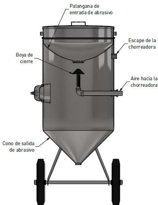
Figura 3 - Elementos principales de los equipos RCH LP. Sección.
